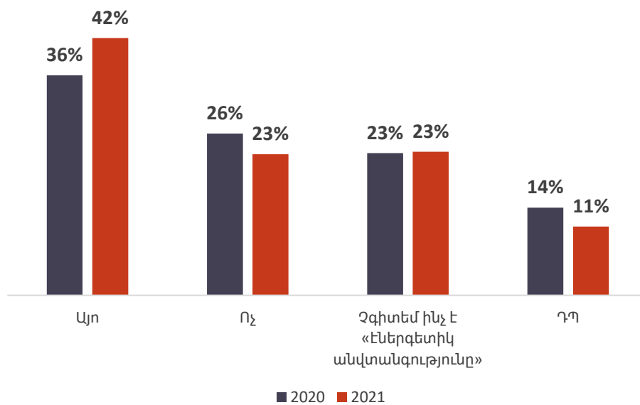
Գծապատկեր 3.10. Ձեր կարծիքով, Հայաստանը էներգետիկ անվտանգության խնդիր ունի՞ n=1100
